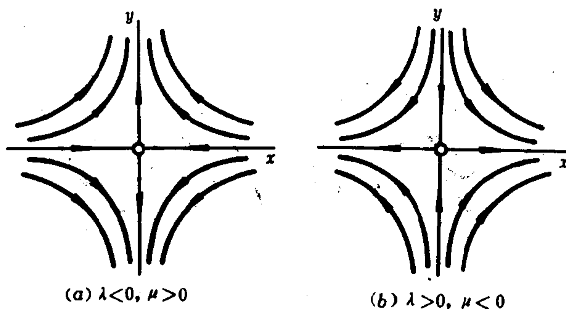
图 8-13 鞍点
