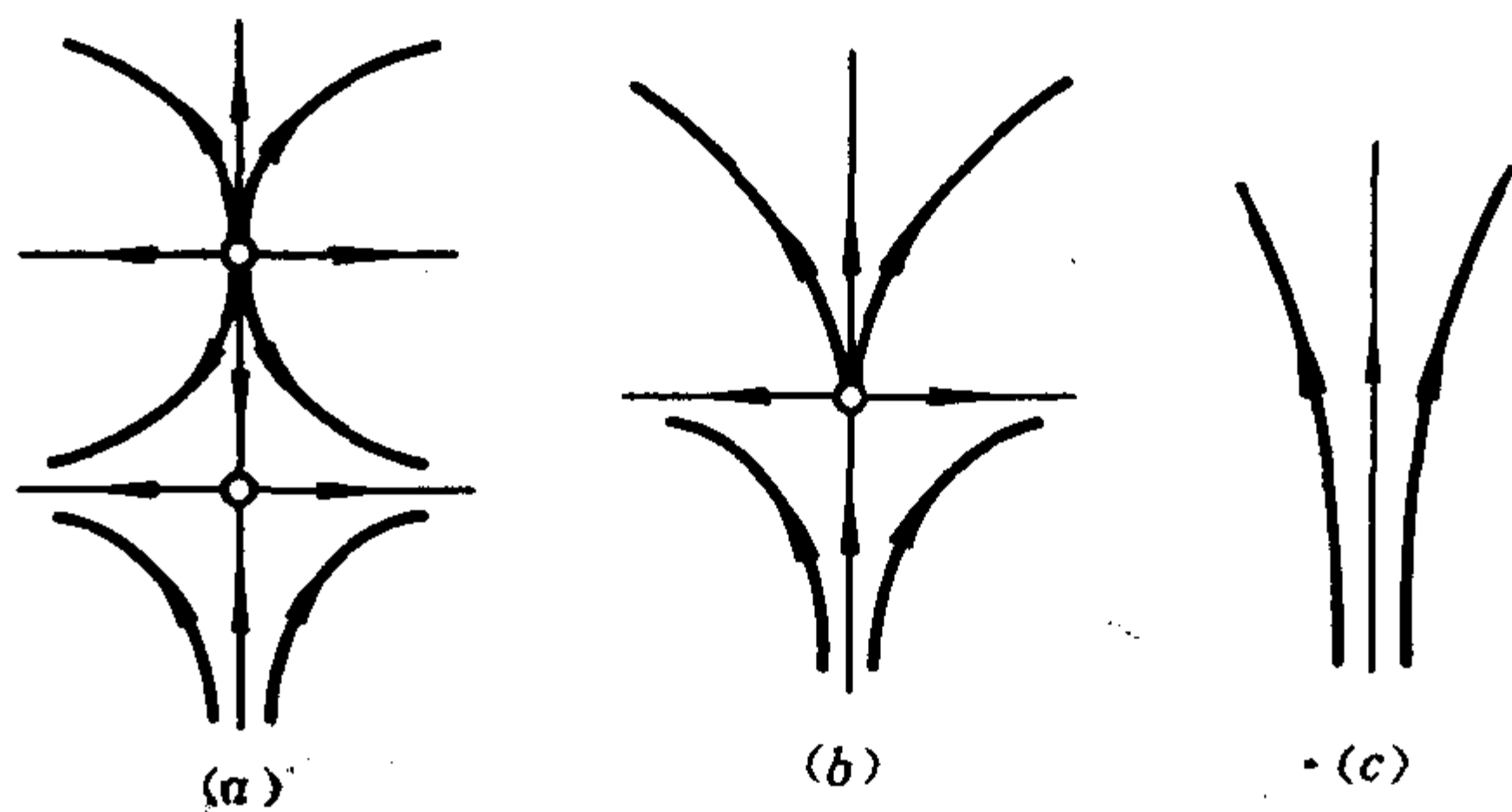
图 8-30 鞍 - 结点分支
