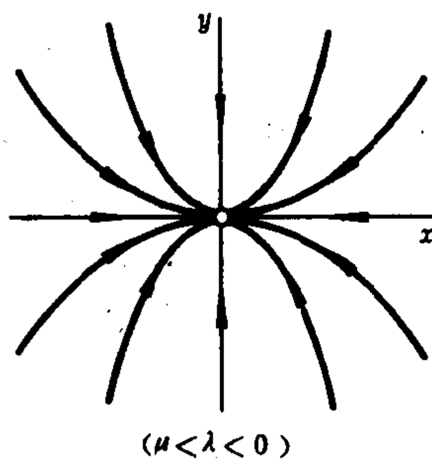
图 8-11 稳定的两向结点
