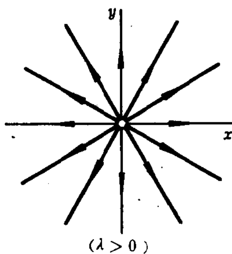
图 8-10 不稳定的星形结点
