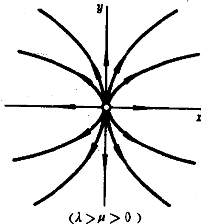
图 8-12 不稳定的两向结点
