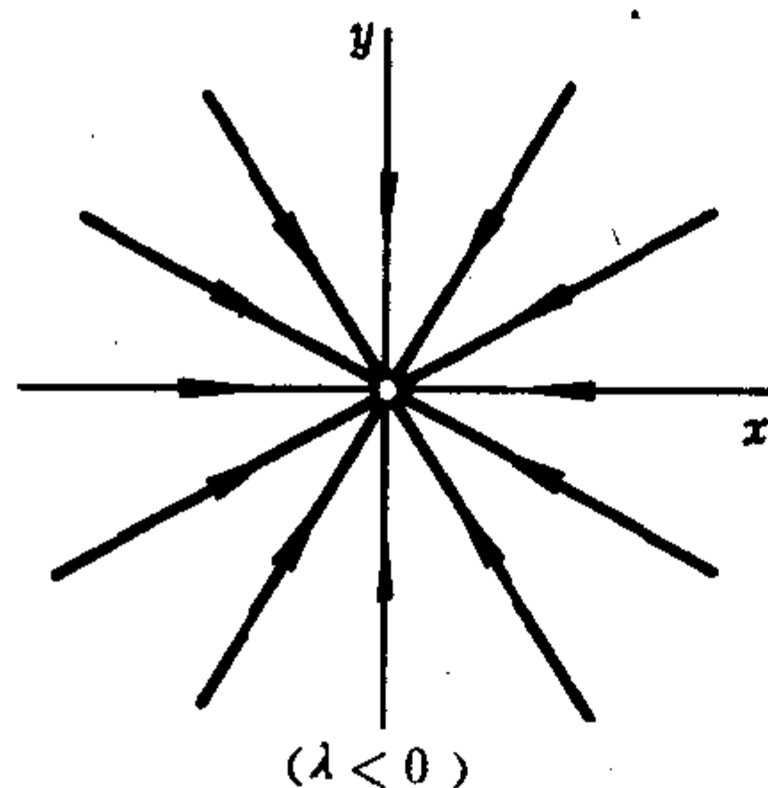
图 8-9 稳定的星形结点
