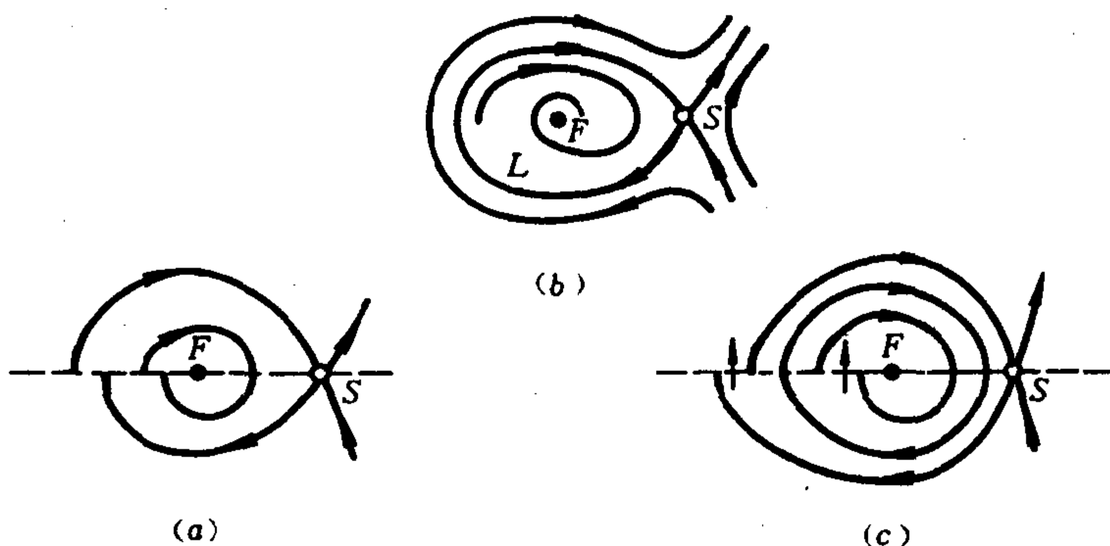
图 8-33 同宿轨线的分支
